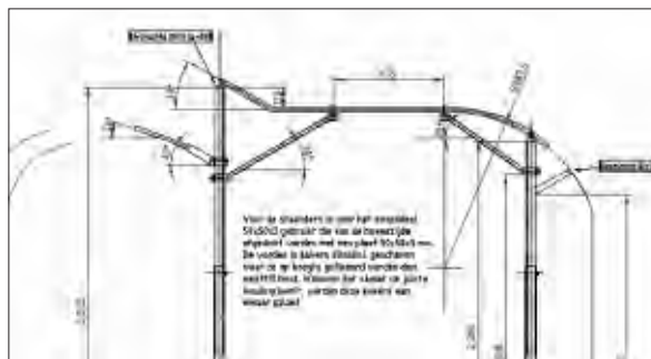
BOUWTEKENING VAN DE DRAAGCONSTRUCTIE VOOR HET SKELET. [ILLUSTRATIE: ROCHUS BIESHEUVEL]
